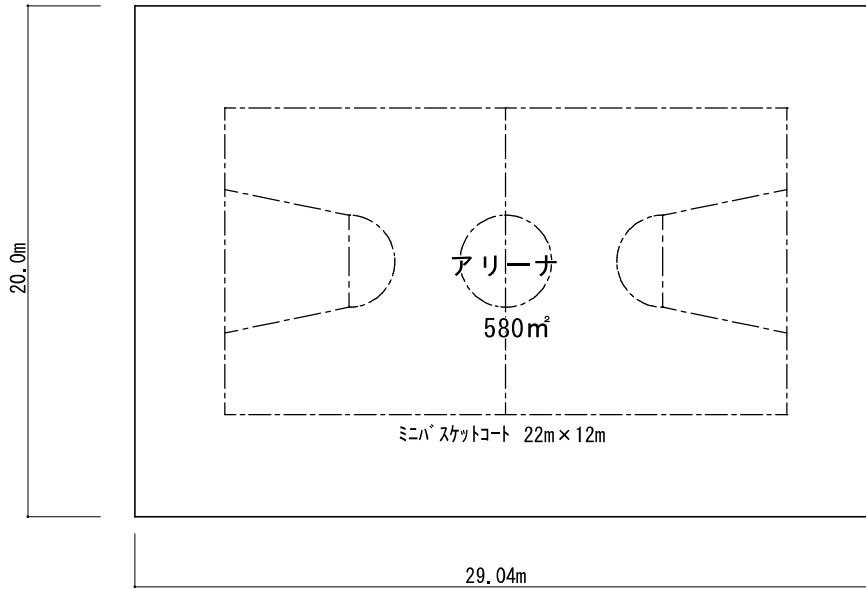
既存体育館アリーナ平面
