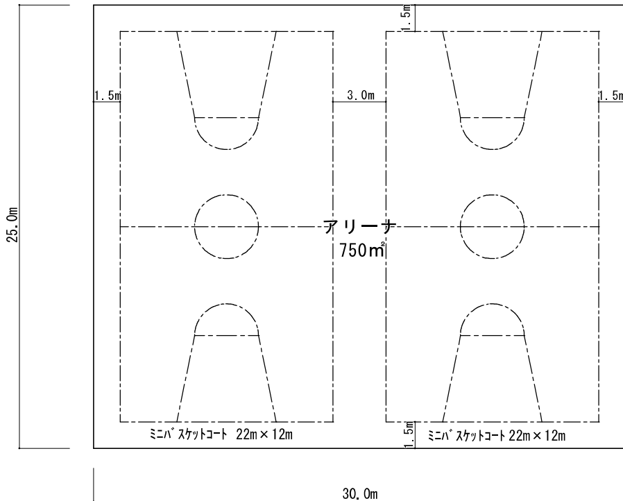
改築体育館アリーナ平面
