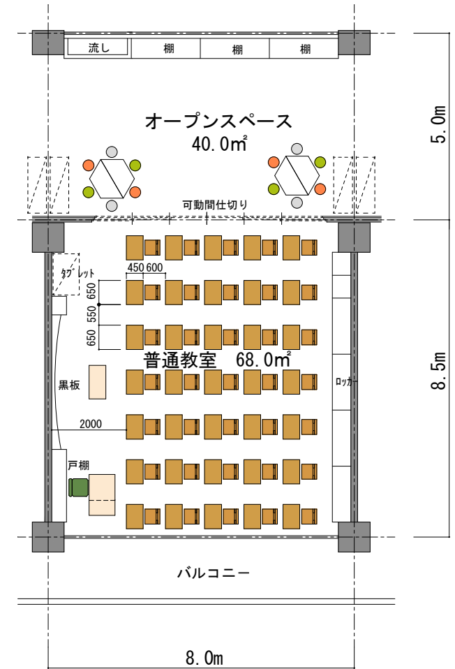
普通教室イメージ図2 (新JIS机 レイアウト 35人)
