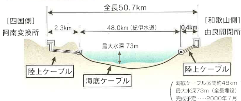
海底ケーブル布設図
