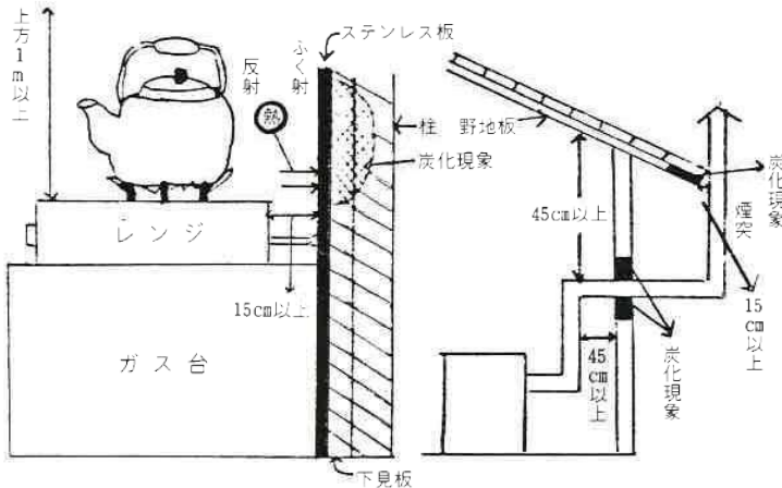
図2 煙突は可燃物より15cm以上の距離をとり、貫通部には眼鏡石(コンクリートや石綿などでできた四角い枠)をはめ込みましょう。
