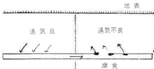
図3 酸素供給程度の異なる2種の土壌にまたがった配管の腐食
