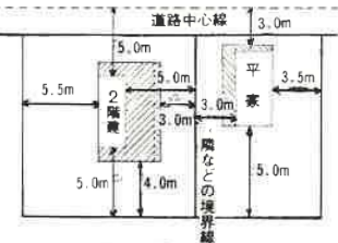
延焼のおそれのある部分を示す
