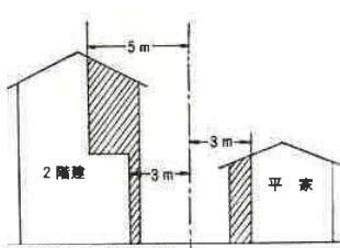
平地境界線（または道路中心線、同一敷地内の2以上の建築物相互の外壁中心線）
