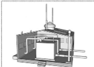
屋内タンク貯蔵所(4)
