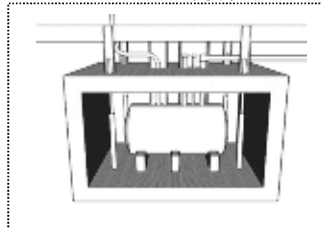
地下タンク貯蔵所(41)
